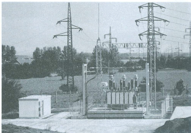
Provizorní napáječ 110/23kV
