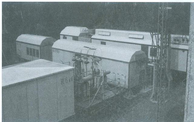
Převozná měnárna 3kV a rozvodna 6kV AC
